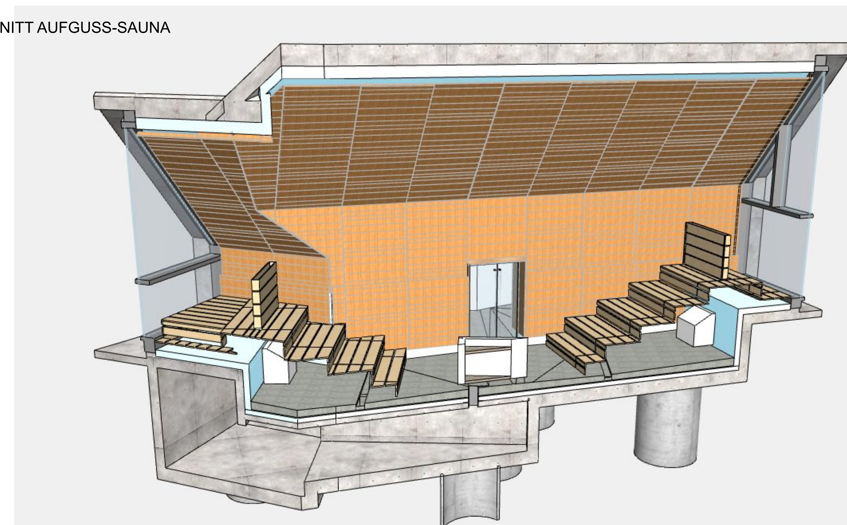
S-14 SCHNITT AUFGUSS-SAUNA 1:20
