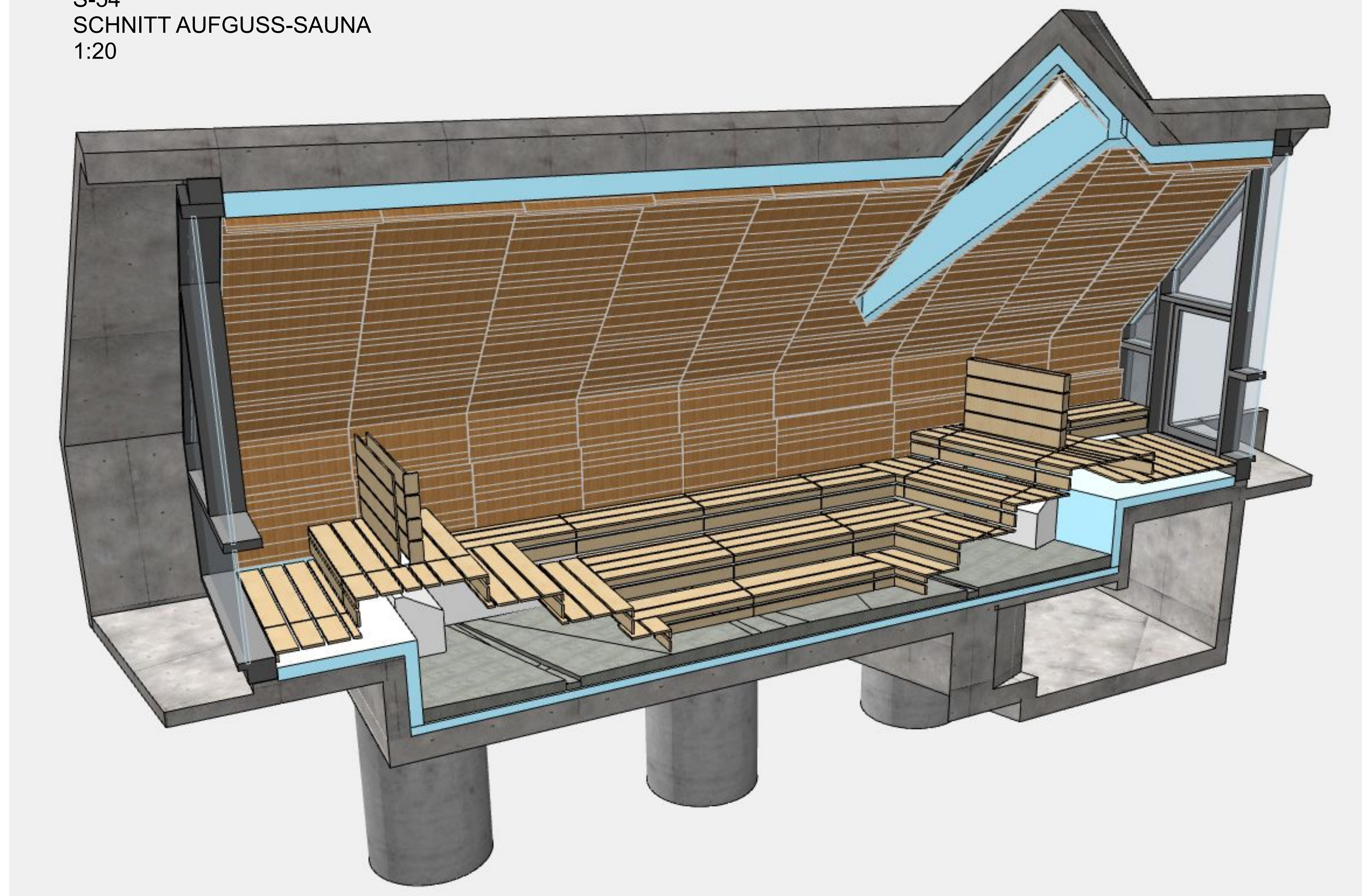
S-17 SCHNITT AUFGUSS-SAUNA 1:20
